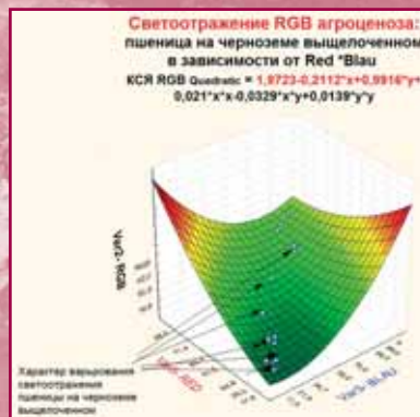
Рис. 1. Светоотражение агроценоза: яровая пшеница на черноземе выщелоченном
