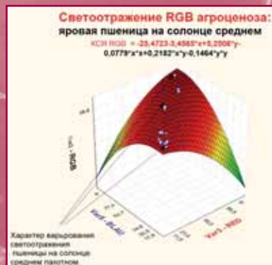
Рис.2. Светоотражение агроценоза: яровая пшеница на солонце среднем
